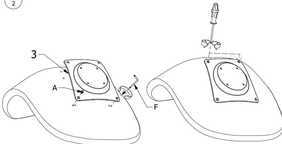
FIG. 2 NB: 402-2090
